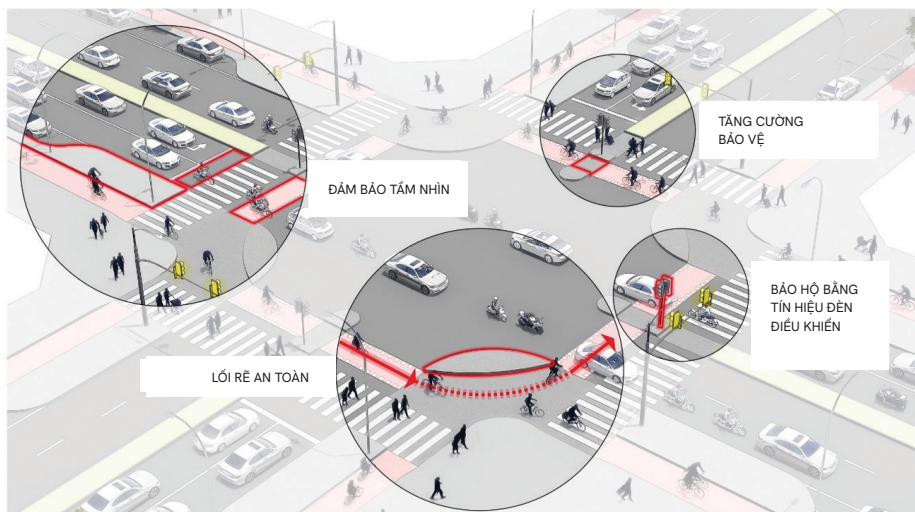
Hình 4.1. Các nguyên tắc chính khi thiết kế nút giao thông cho xe đạp (Nguồn: WRI, 2021)
